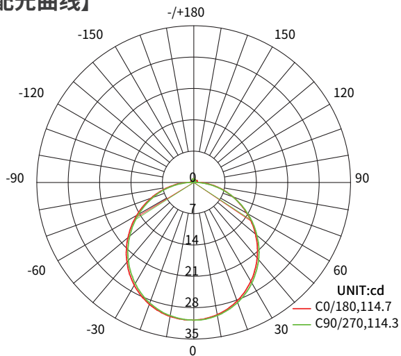
配光曲线
